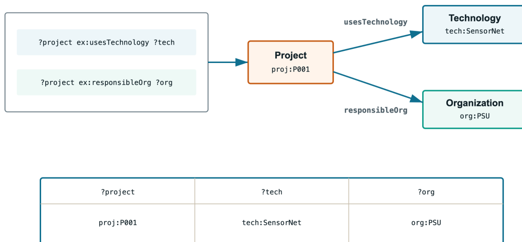
ภาพที่ 4.2: การใช้ตัวแปรร่วมกันเป็นจุดเชื่อมและสร้าง binding ใน SPARQL
