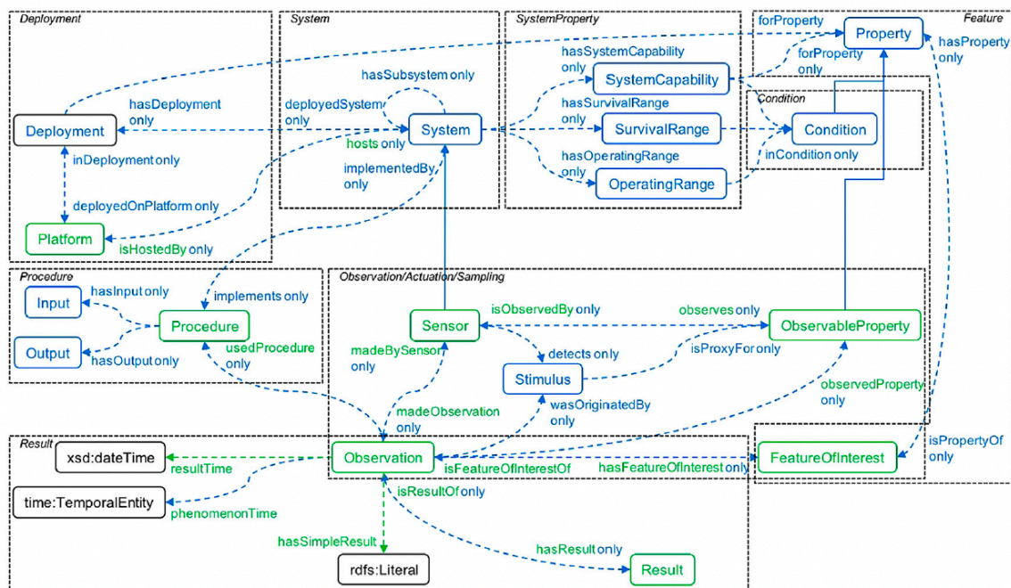
ภาพที่ 6.1: องค์ประกอบของ SSN/SOSA ที่ใช้เป็นฐานสำหรับอธิบาย Sensor, Observation และ Result (ที่มา: Angsuchotmetee et al., 2020, ภาพที่ 3)
