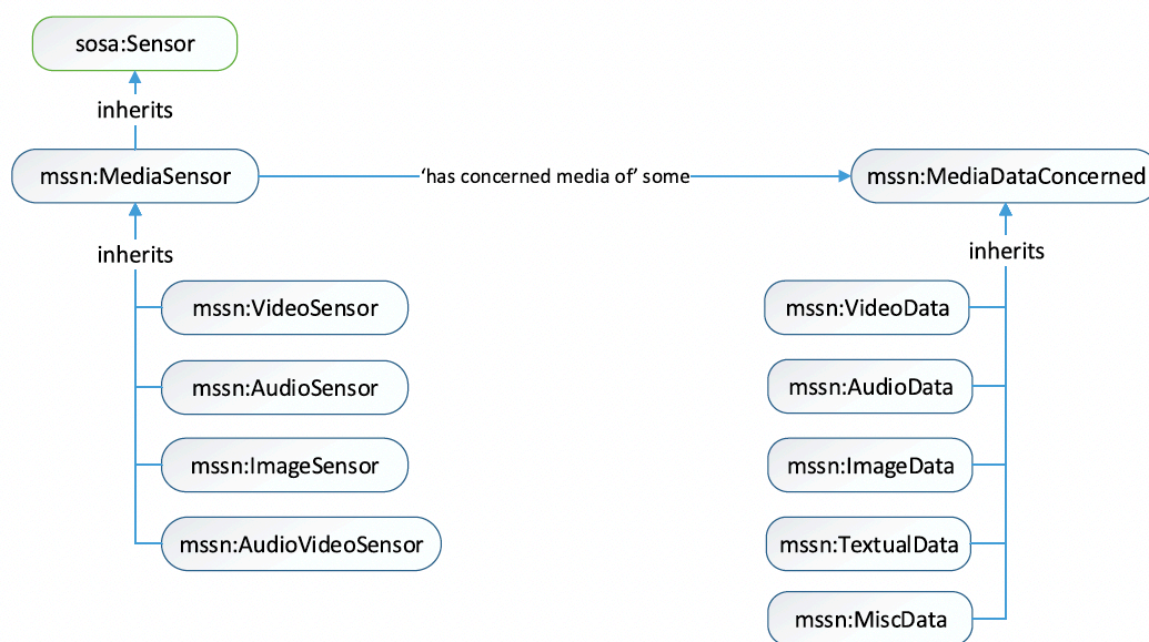
ภาพที่ 6.2: การขยายชนิด Media Sensor และชนิดข้อมูลสื่อใน MSSN-Onto (ที่มา: Angsuchotmetee et al., 2020, ภาพที่ 4)
