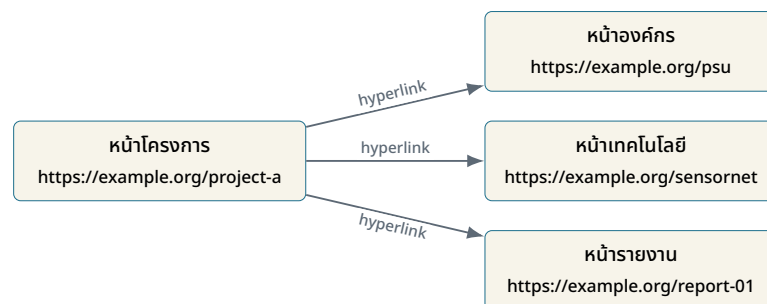
ภาพที่ 1.1: เว็บทั่วไปในฐานะเครือข่ายของเอกสารที่เชื่อมกันด้วย Hyperlink
