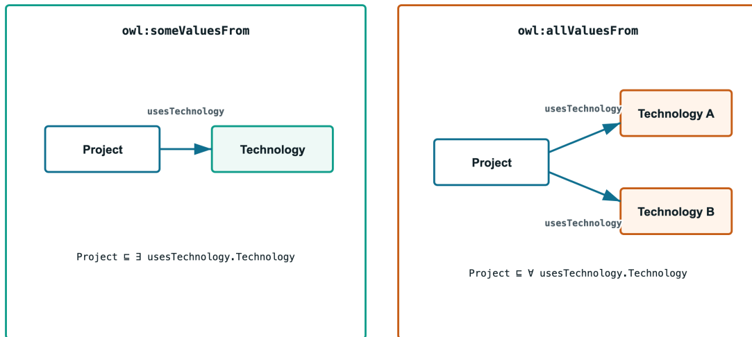
ภาพที่ 3.2: ความต่างระหว่าง owl:someValuesFrom และ owl:allValuesFrom
