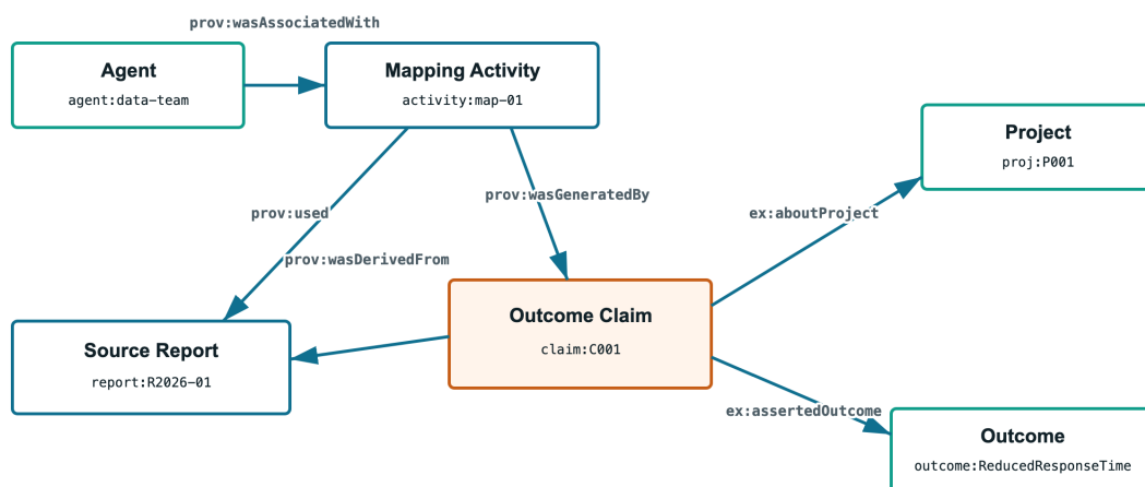
ภาพที่ 9.1: เส้นทาง Provenance ระดับ Claim จากข้อสรุปกลับไปยังรายงานและกิจกรรมที่สร้างข้อมูล
