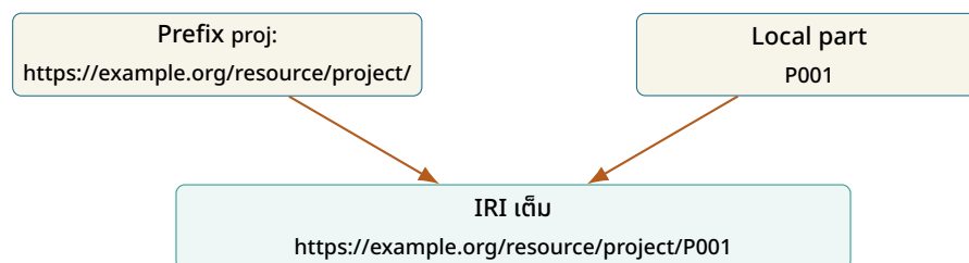
ภาพที่ 1.4: การขยาย Prefix และ Local Part กลับเป็น IRI เต็ม
