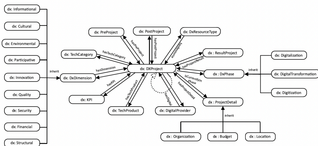
ภาพที่ 6.4: โครงสร้างแกนของ Dx-Onto ที่เชื่อมโครงการกับ Phase, Dimension, Resource และรายละเอียดที่เกี่ยวข้อง (ที่มา: ภาพที่ 3 ในต้นฉบับผู้เขียนของงาน Ben-arlee and Angsuchotmetee, 2026)
