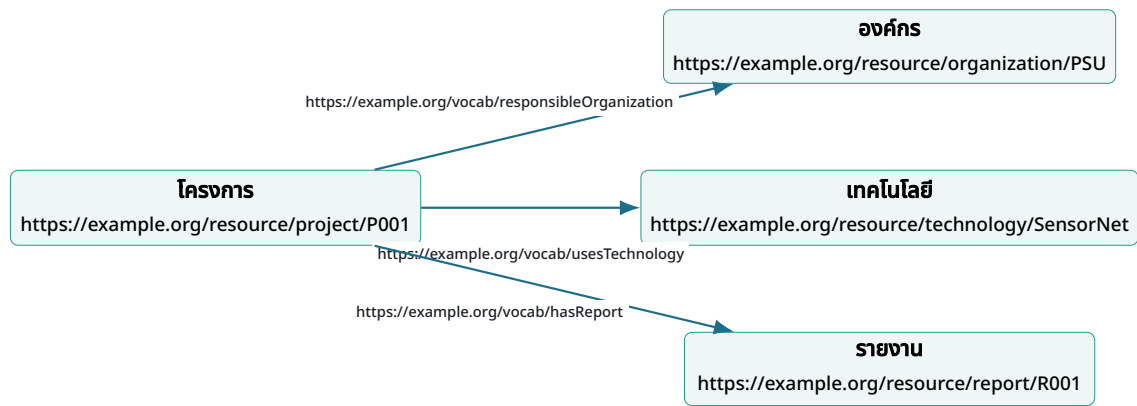
ภาพที่ 1.2: กราฟเชิงความหมายที่ Resource และความสัมพันธ์มี IRI ชัดเจน
