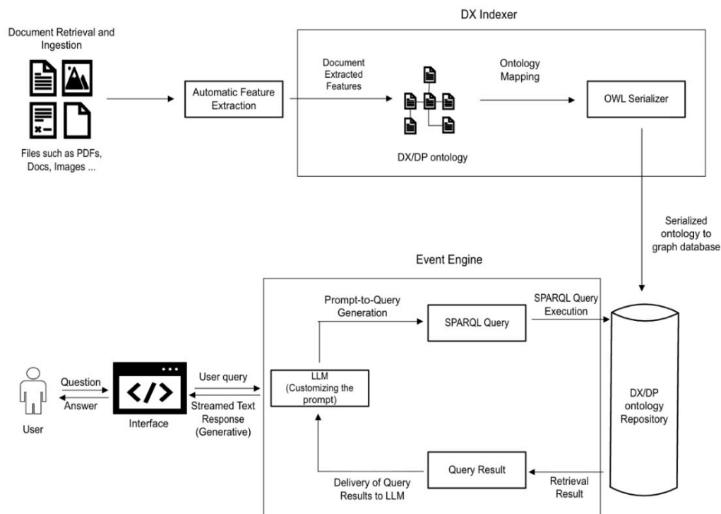
ภาพที่ 10.2: แนวทาง Hybrid LLM-Ontology ที่แบ่ง Ontology Indexing ออกจาก Semantic Recall
