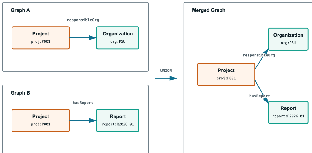
ภาพที่ 2.2: การรวม RDF Graph จากสองแหล่งด้วย IRI ของโครงการเดียวกัน
