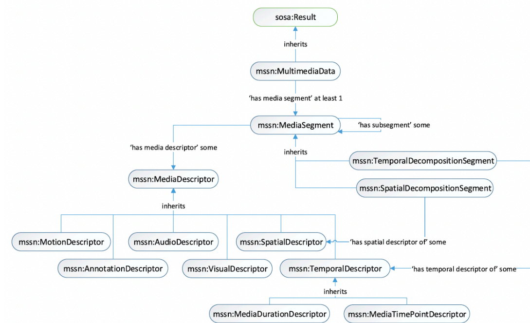
ภาพที่ 6.3: การออกแบบ Multimedia Data, Media Segment และ Media Descriptor ใน MSSN-Onto (ที่มา: Angsuchotmetee et al., 2020, ภาพที่ 6)
