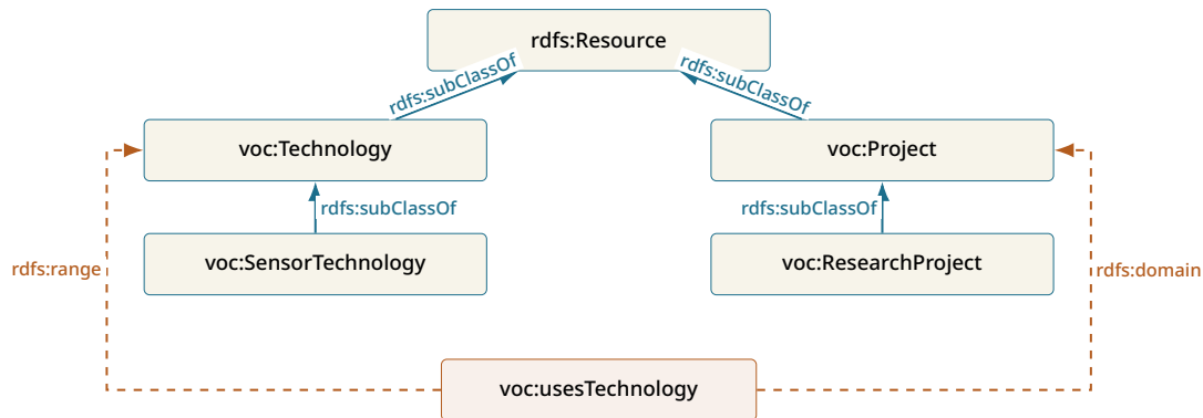
RDFS อธิบายลำดับชั้นและขอบเขตความหมายของคำศัพท์
